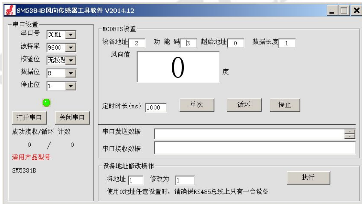
图 3 软件界面
