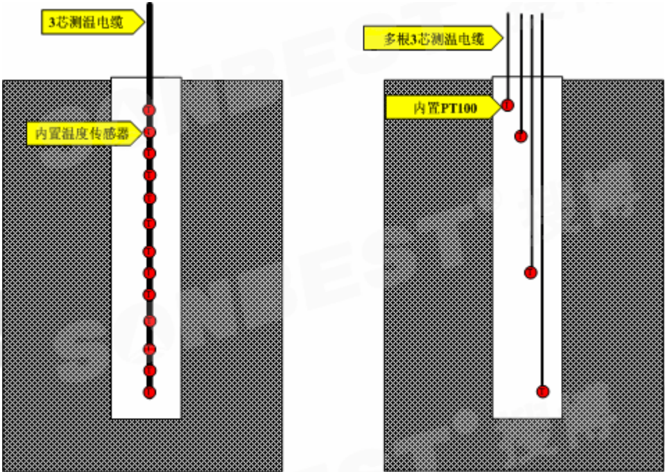
布线方式对比
