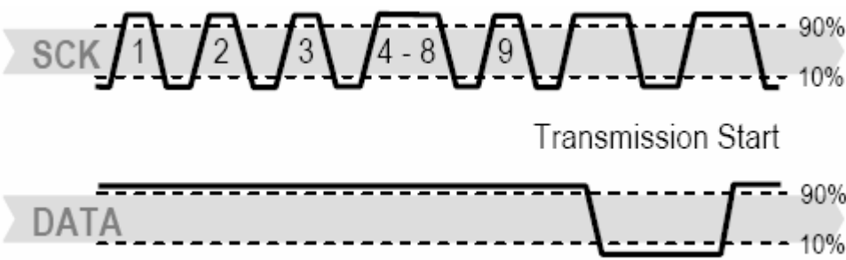
图 8 通讯复位时序
